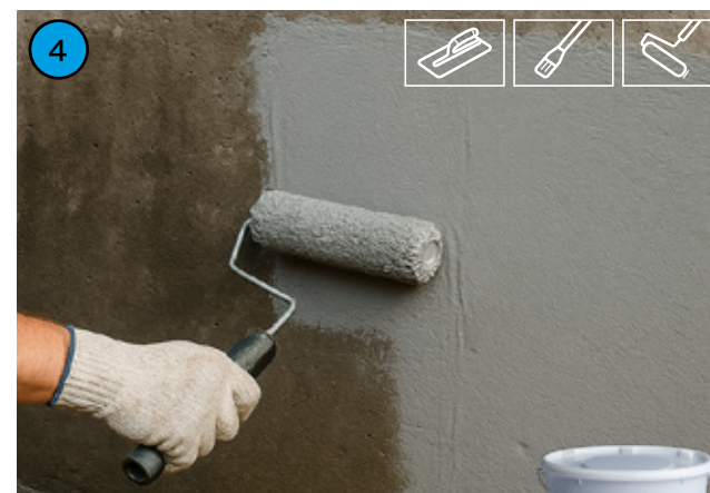
Applicazione di BETONGUAINA BASEMENT in due mani a rullo, pennello o frattazzo.
