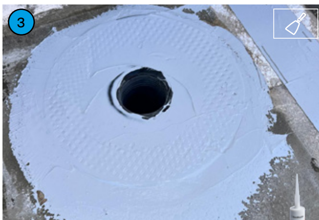
3 Posizionamento degli scarichi e sigillatura con BETONSEAL MS 2.0 .
