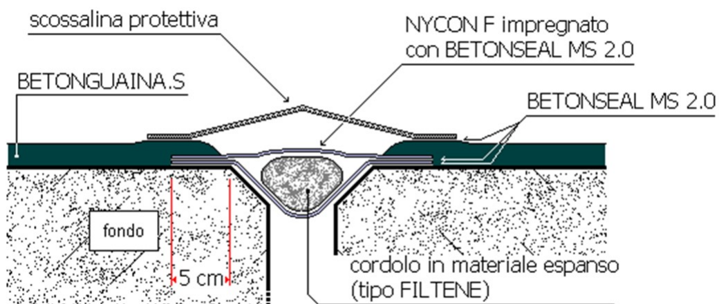
Figura 8 - Realizzazione di giunti di dilatazione strutturali.
