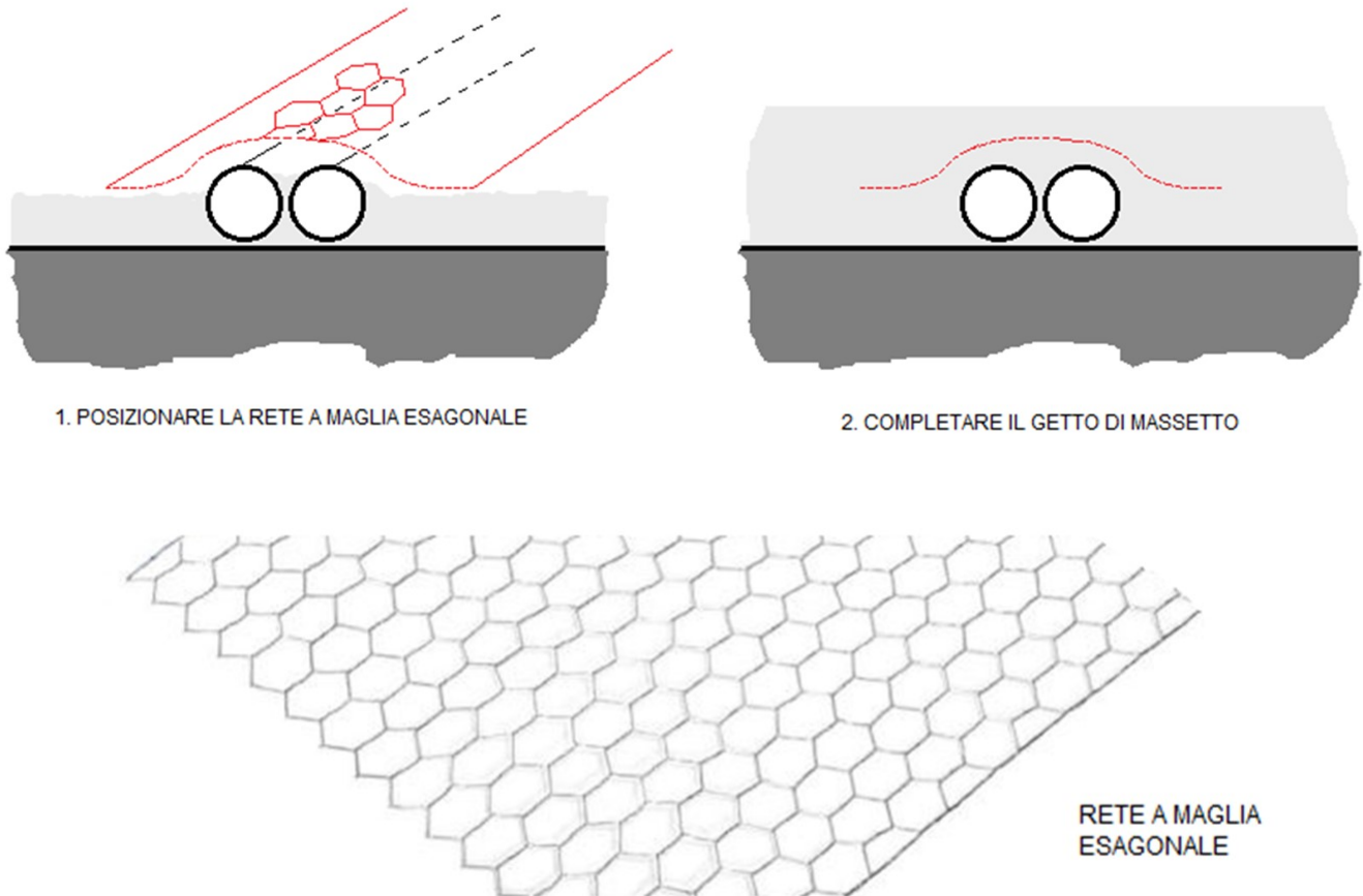
Fig. 3: inserimento della rete di rinforzo sopra tubazioni o canalizzazioni
